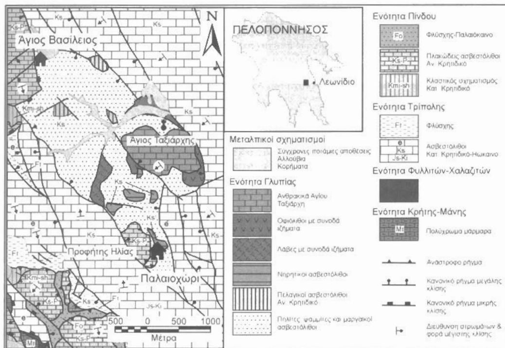
Εικ. 1: Γεωλογικός χάρτης της περιοχής μελέτης. Διακρίνεται η επιφανειακή εξάπλωση της ενότητας Γλυπίας με τις σημαντικότερες και μεγαλύτερες εμφανίσεις των διαφόρων εξωτικών τεμαχίων μέσα στη κύρια μάζα της. Fig. 1: Geological map of the study area. The main occurrences of some exotic blocks within the Glypia unit, are indicated.
