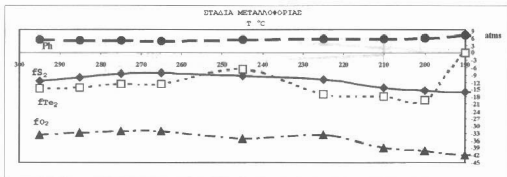
Εικόνα 7. Συμπερασματικό διάγραμμα μεταβολής των φυσικοχημικών παραμέτρων του μεταλλοφόρου ρευστού κατά την εξέλιξη της μεταλλοφορίας της περιοχής Πανόρμου-Λαρδιάδων, στην Τήνο. 1. f_{S_2} : Διαφυγότητα Θείου, 2. f_{O_2} : Διαφυγότητα Οξυγόνου, 3. f_{Te_2} : Διαφυγότητα Τελλουρίου.
