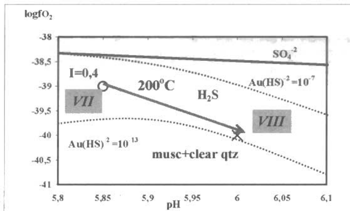
Εικόνα 6. Διάγραμμα f_{O_2} και Ph , για τους 200^\circ C και για τα Στάδια VII, VIII. 1. musc : Μοσχοβίτης, 2. Clear qtz : Γκρίζος Χαλαζίας, 3. H_2S : Υδρόθειο.
