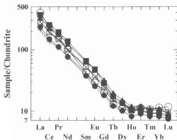
Ψηφιακή Βιβλιοθήκη "Θεόφραστος" - Τμήμα Γεωλογίας, Α.Π.Θ. Figure 4. Chondrite-normalized REE pattern of Sandúklú lavas.
