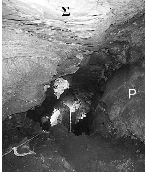
Σχήμα 6. Το κεκλιμένο σπήλαιο ανατολικά από τη θέση Γεράκι. Διακρίνεται η κατοπτρική επιφάνεια του ρήγματος (P) με στοιχεία 71^{\circ}/038^{\circ} , αλλά και η στρώση (Σ) των τριαδικών ασβεστολίθων «του Δρυμού».
